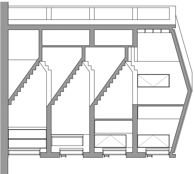
05 SEZIONE (m 2 )
