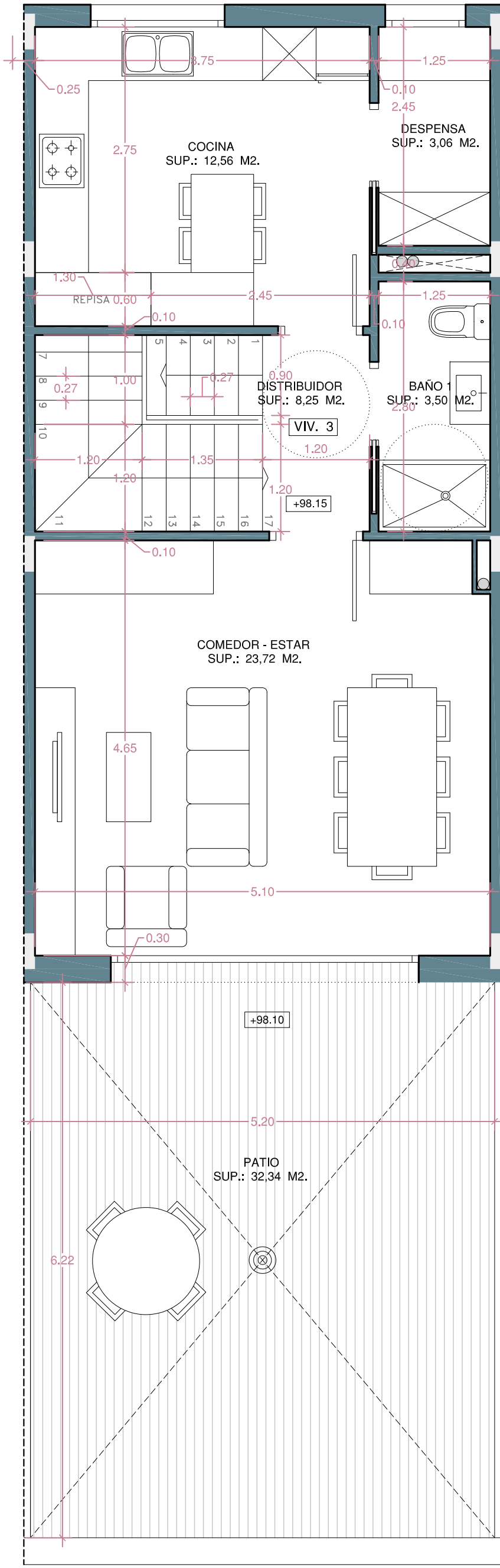
PLANTA PRIMERA - ZONA DIA
