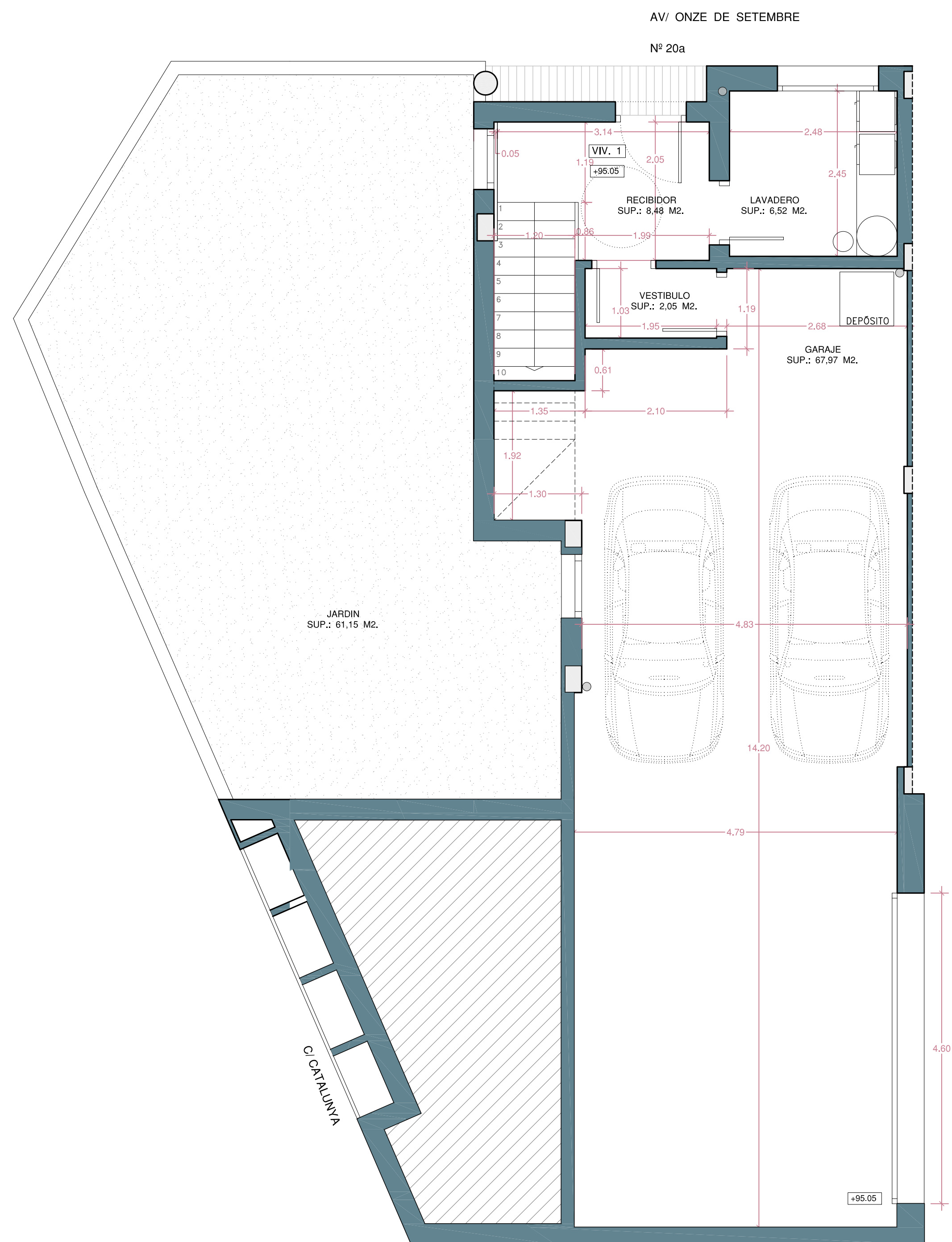
PLANTA BAJA - GARAJE Y ACCESO A VIVIENDA
