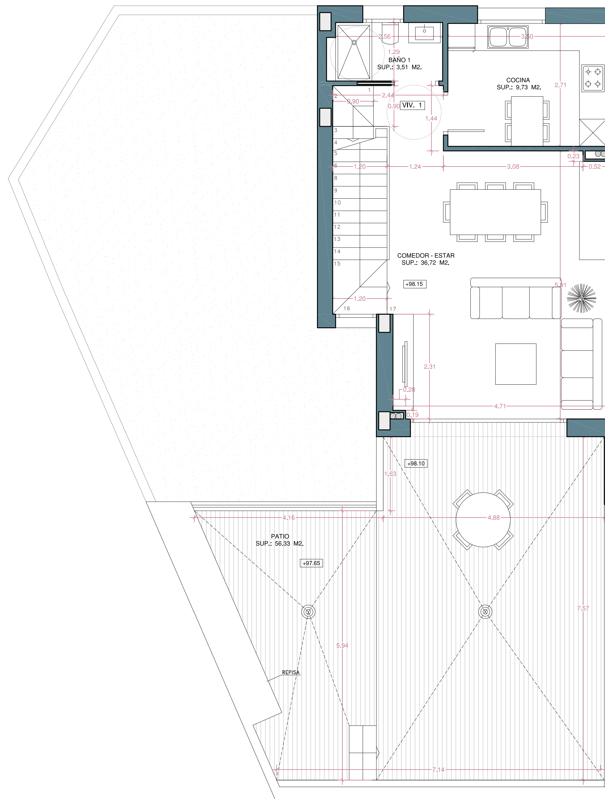
PLANTA PRIMERA - ZONA DIA
