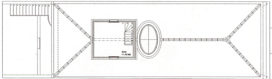
MANSARDA/COBERTURA
