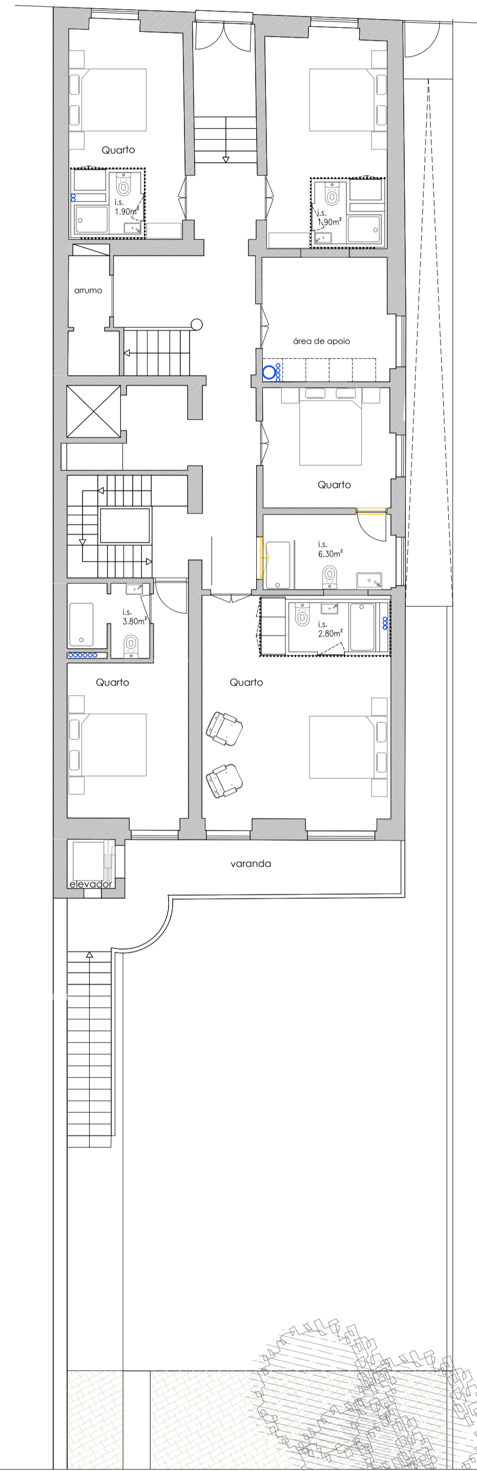
planta do rés do chão
