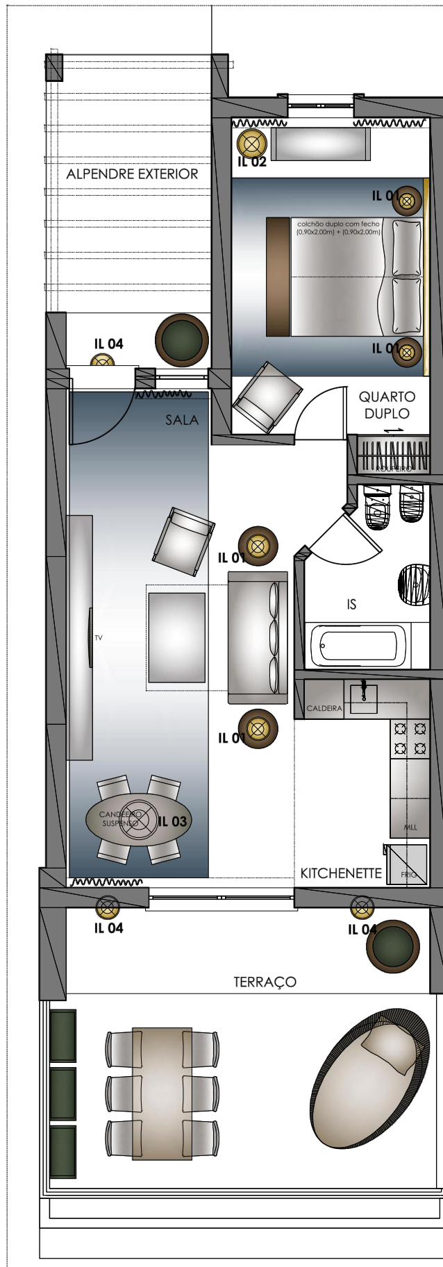
PLANTA PISO TIPO
