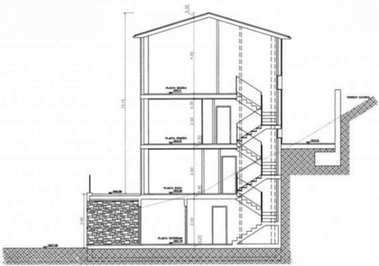
SECCION AA
