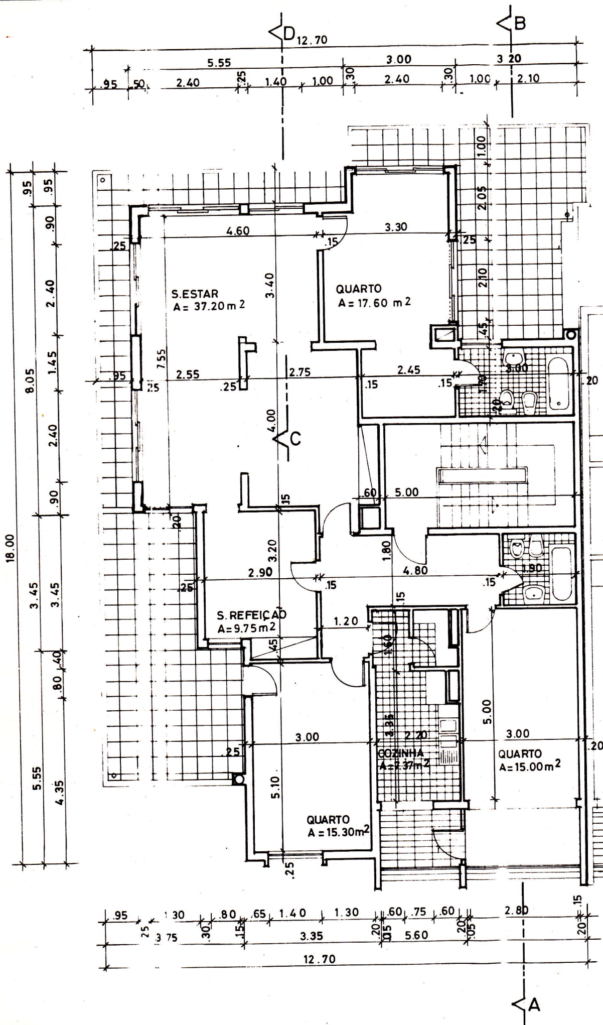
PLANTA DO 3 ANDAR
