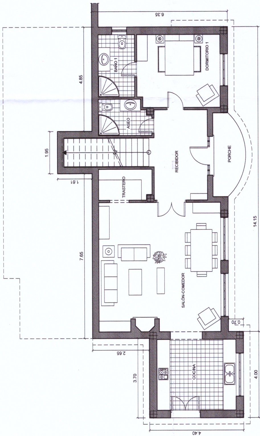
PLANTA BAJA
