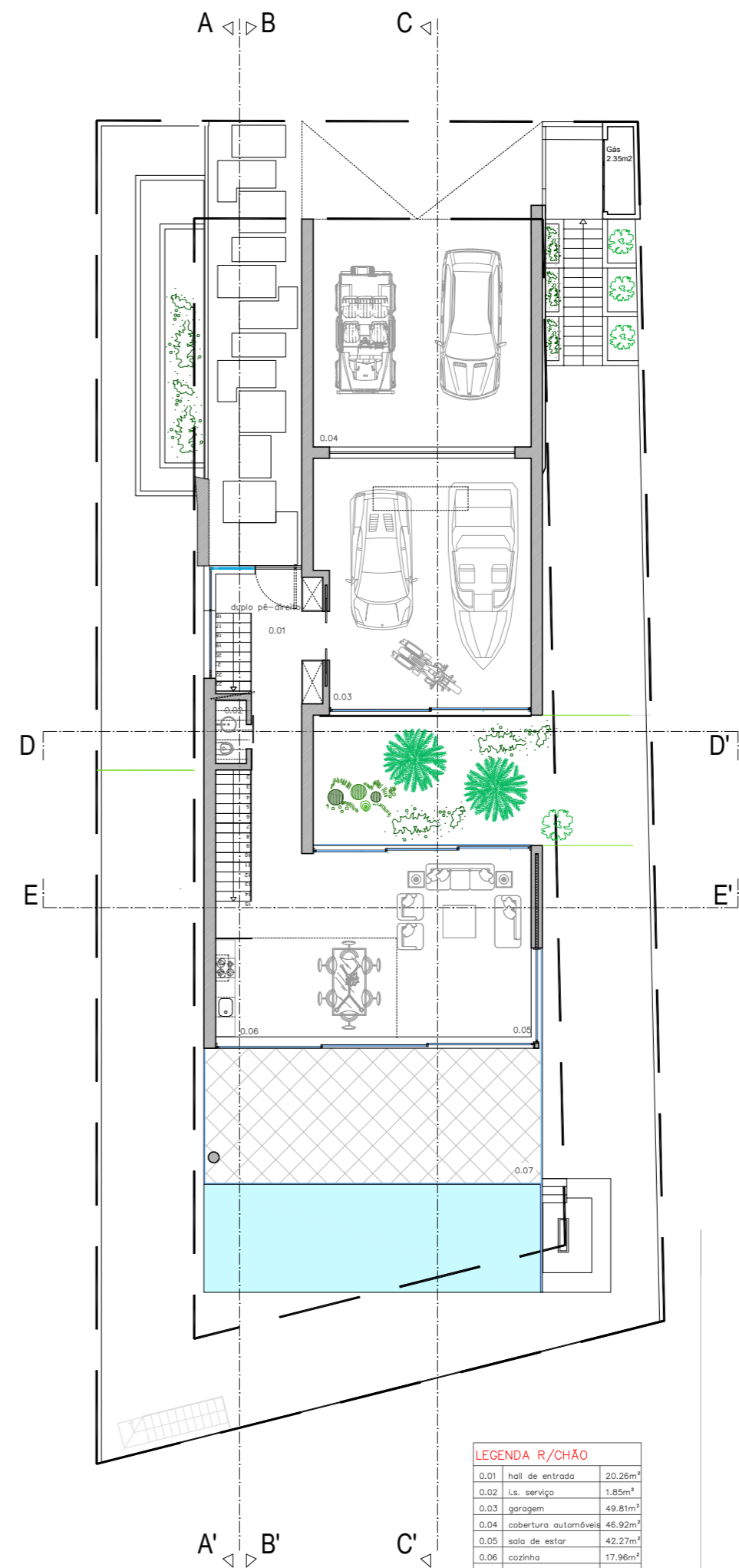
PLANTA R/CHÃO
