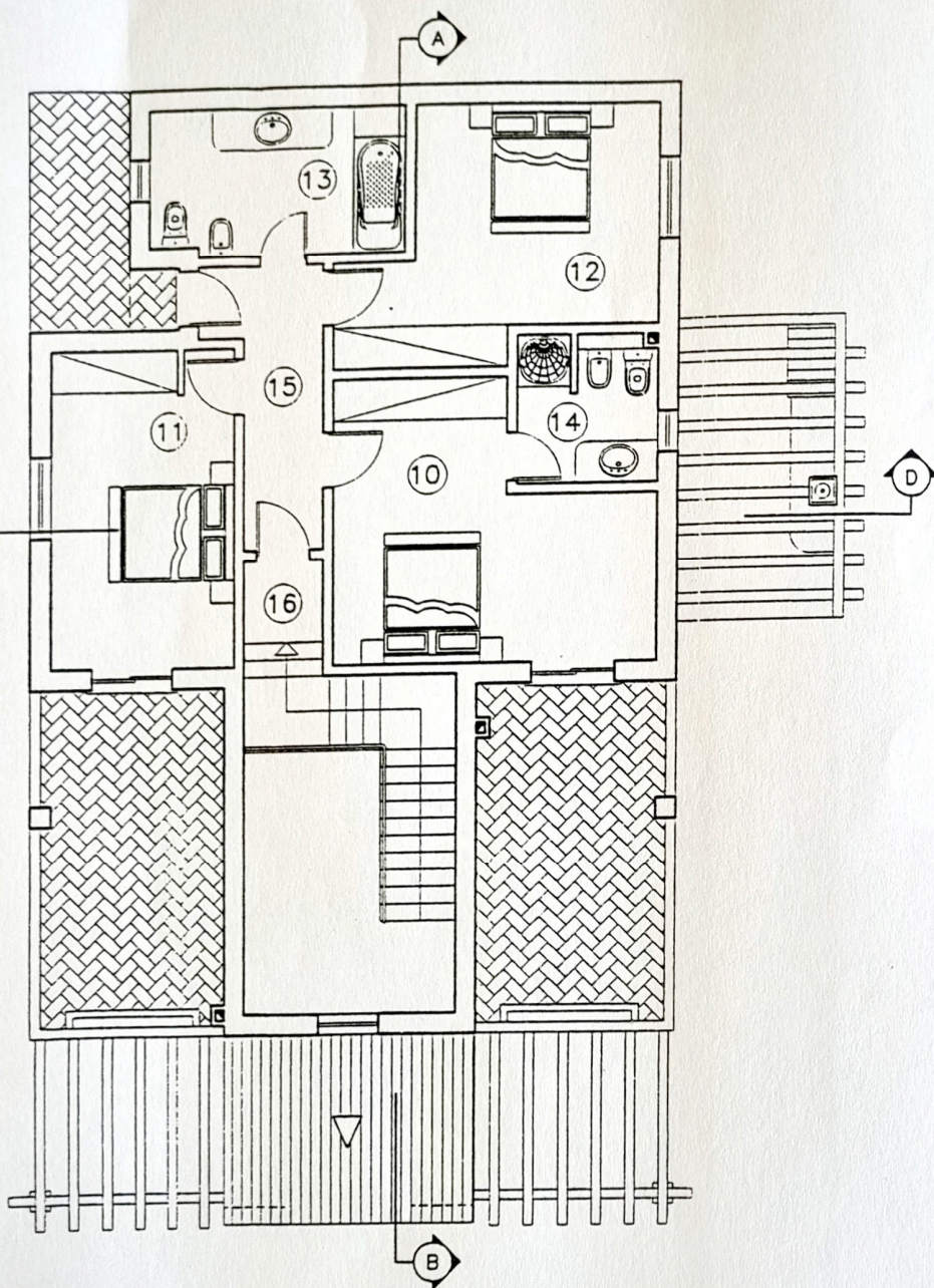
PLANTA DO 1º ANDAR
