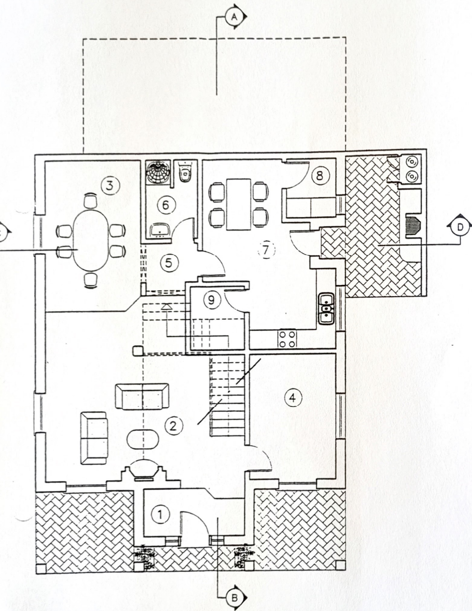
PLANTA DO R/C
