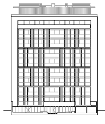
ALÇADO TARDOZ REAR FACADE FAÇADE ARRIÈRE
