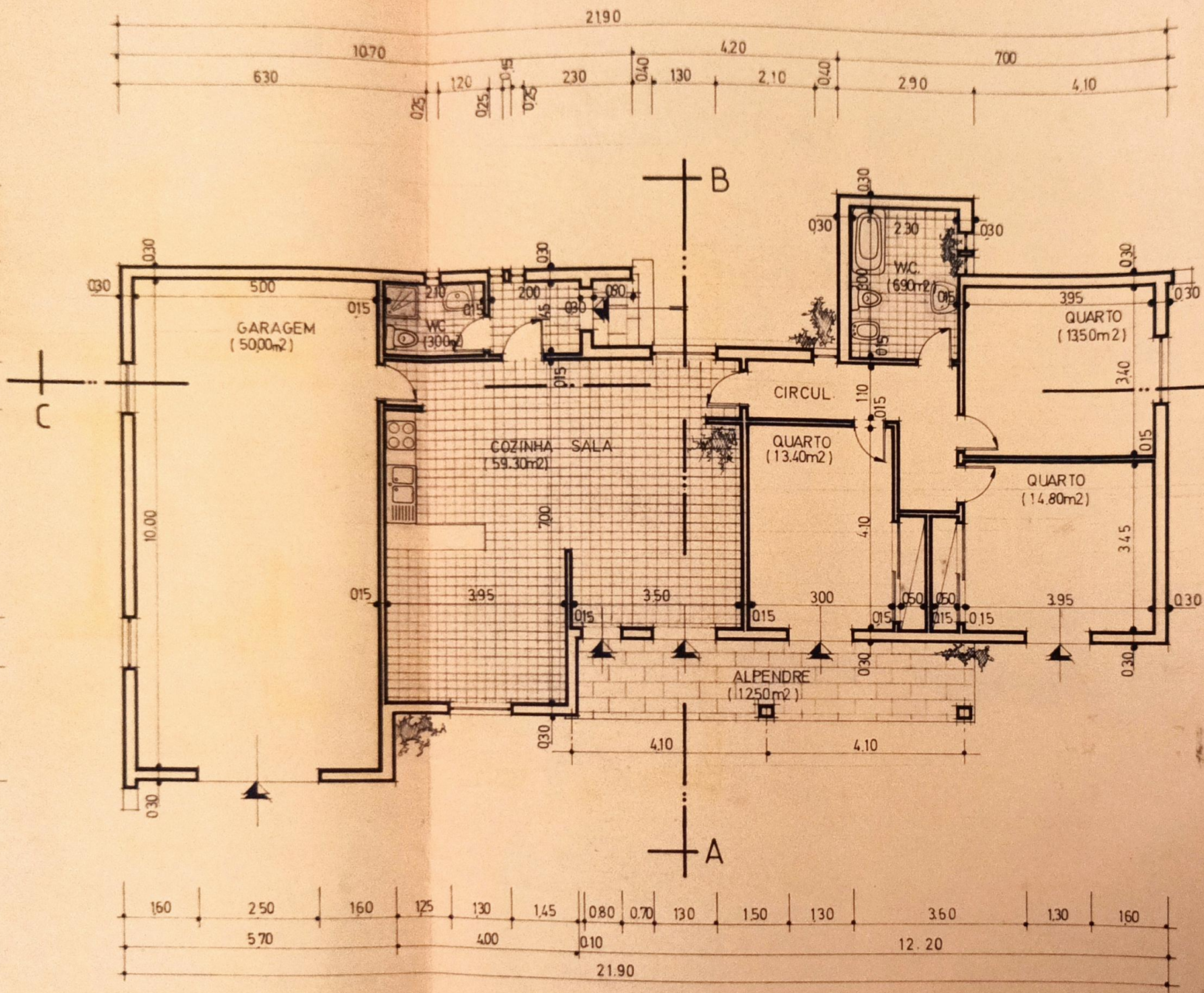
PLANTA DO PISO
