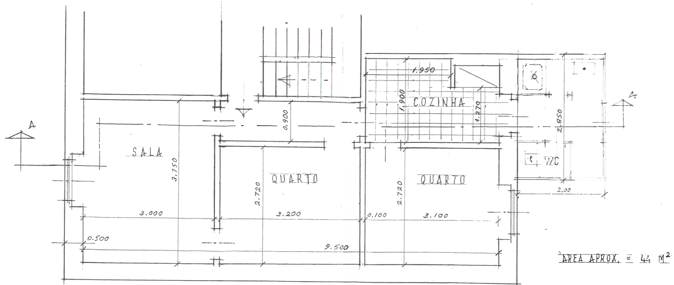
PLANTA
