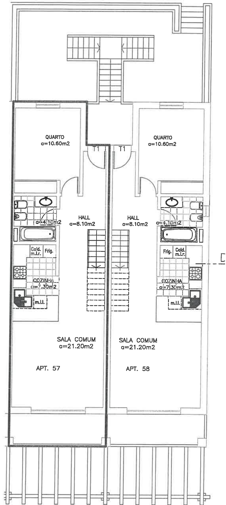
PLANTA DO PISO 1
