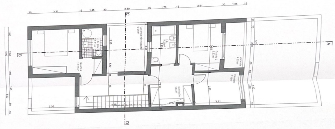
Planta do 1º andar
