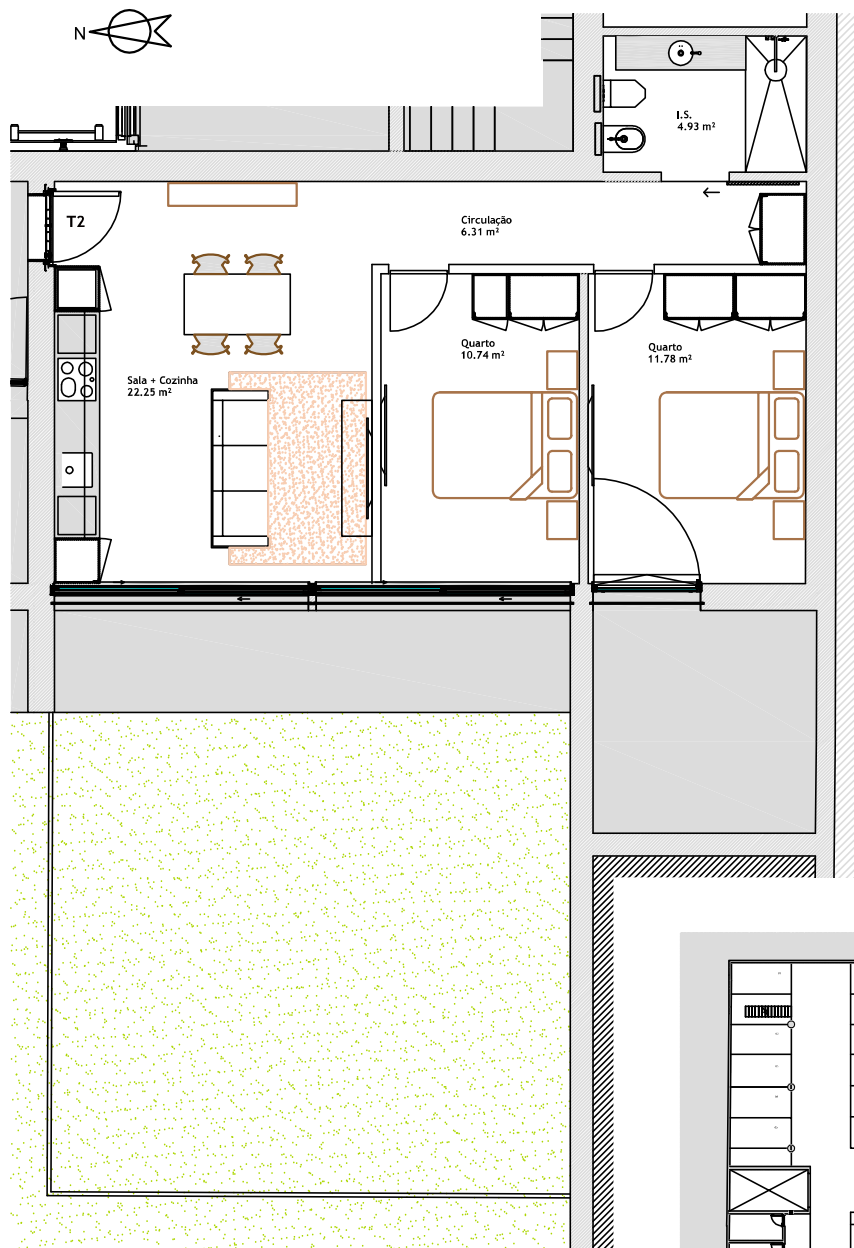
Planta da Fração
