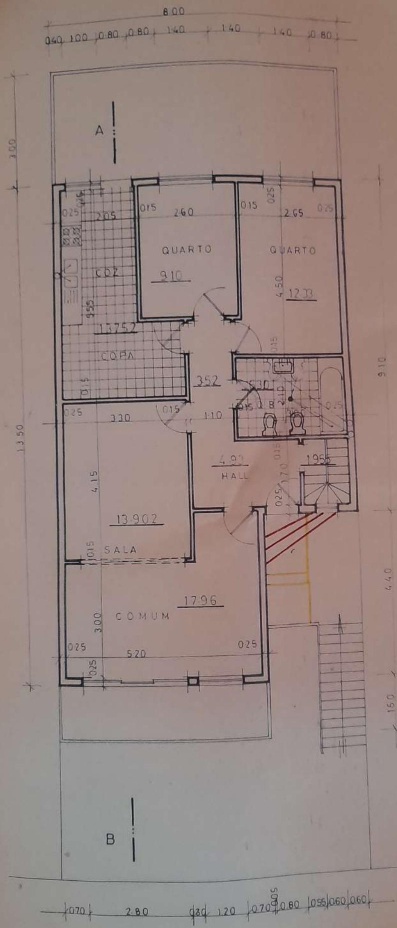
PLANTA DO 1º ANDAR
