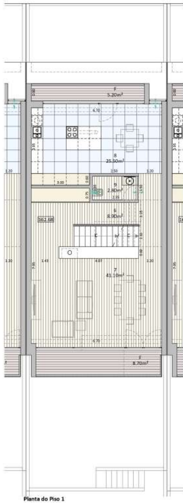
Planta do Piso 1
