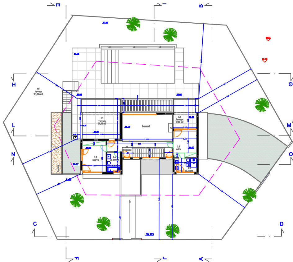
PLANTA PISO 2 - 1º Andar
