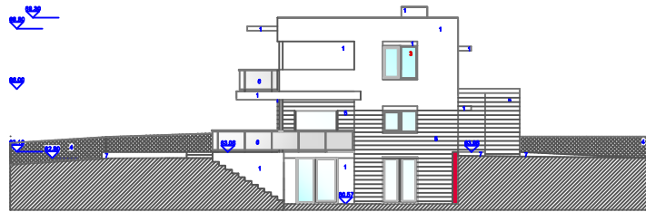
CORTE EF - ALÇADO SUL
