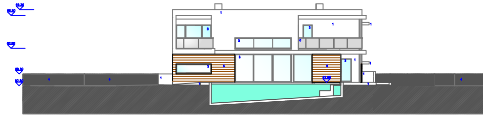
CORTE GH - ALÇADO
