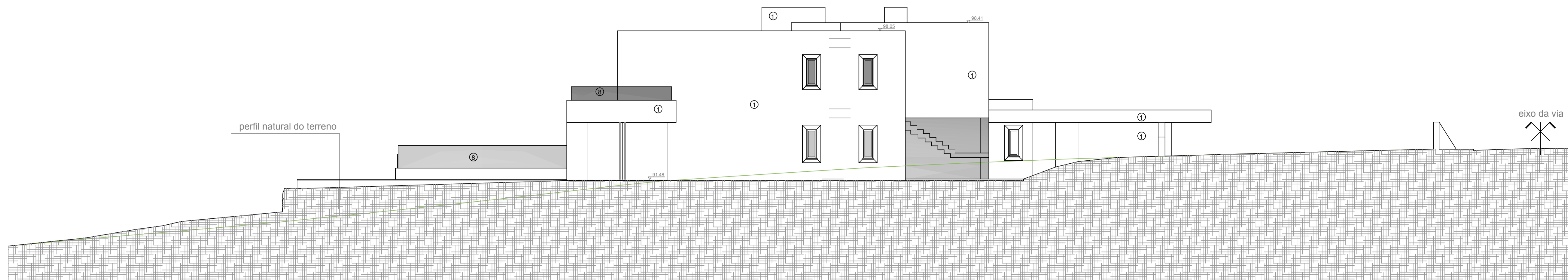
ALÇADO NORTE
