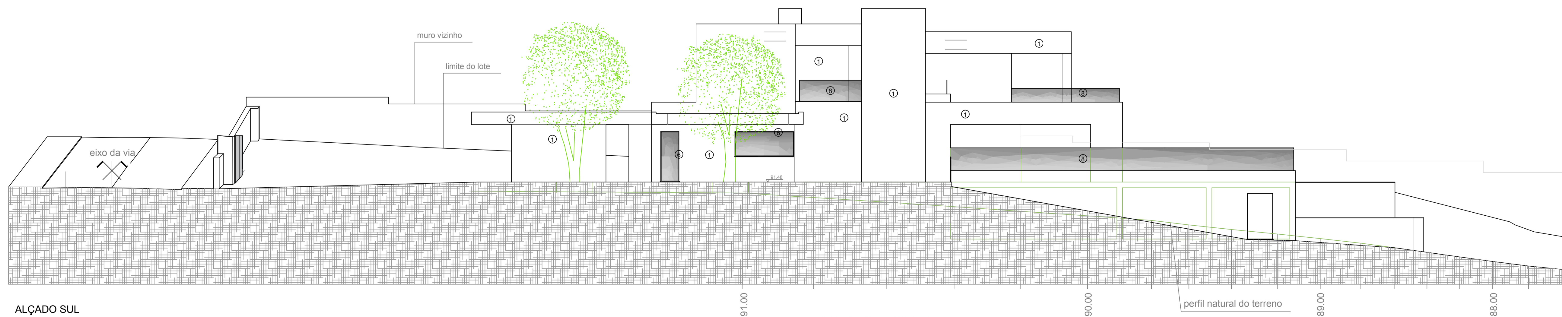
ALÇADO SUL
