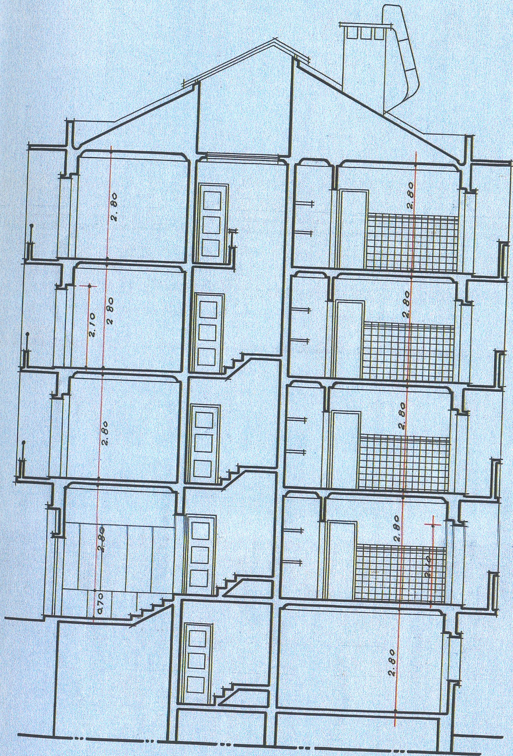
CORTE A~B
