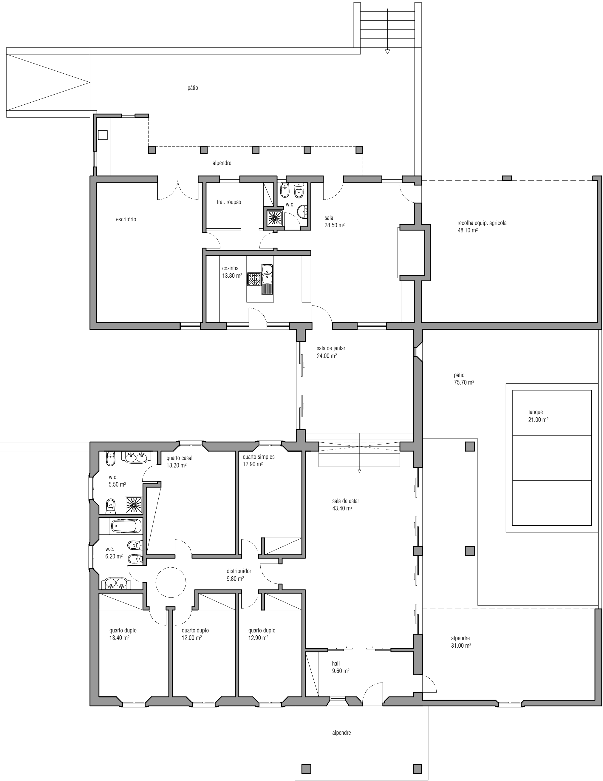
planta habitação
