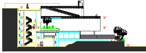
CORTE DD
