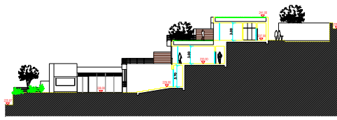
CORTE BB
