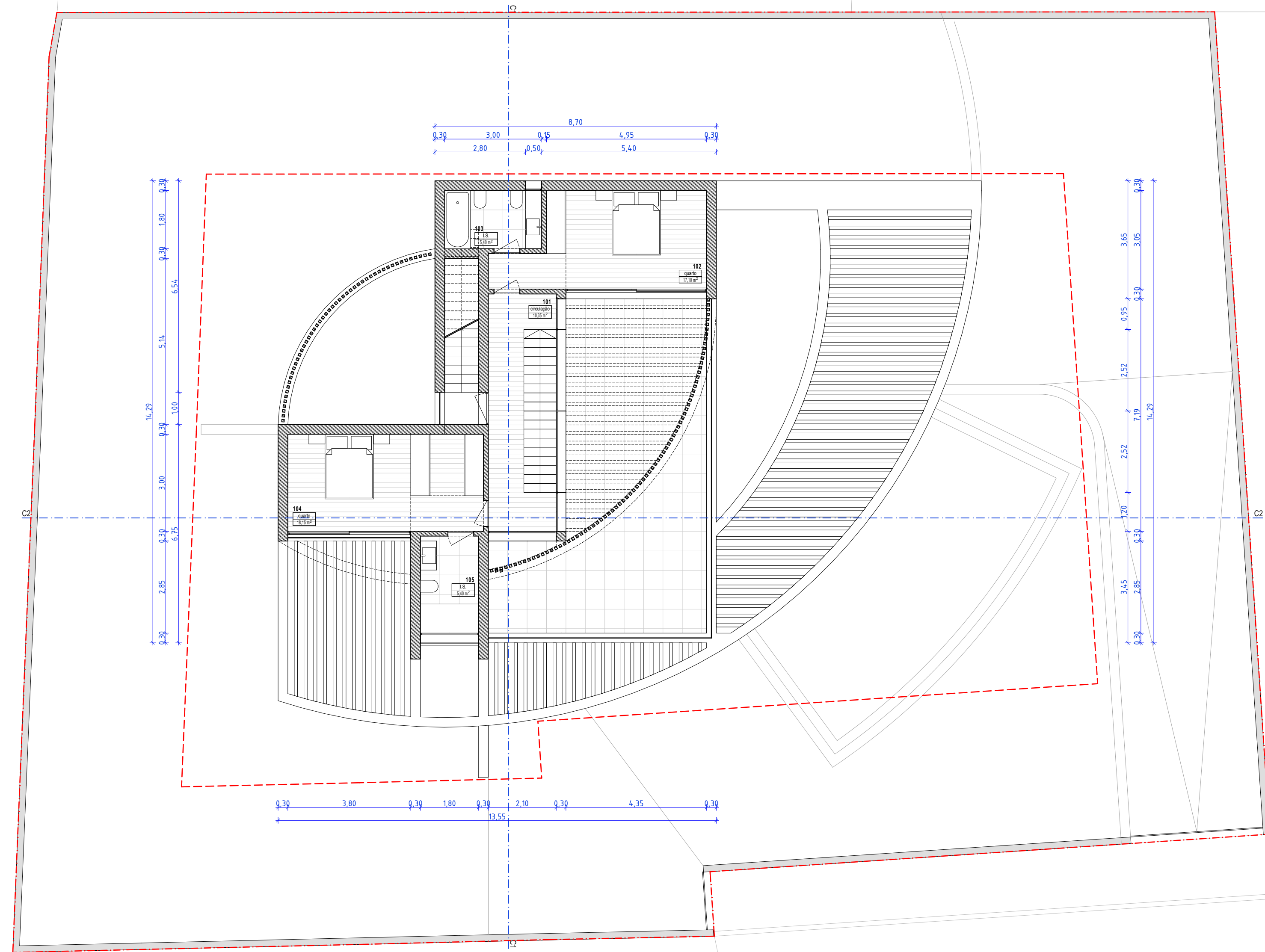
Planta do Piso 1
