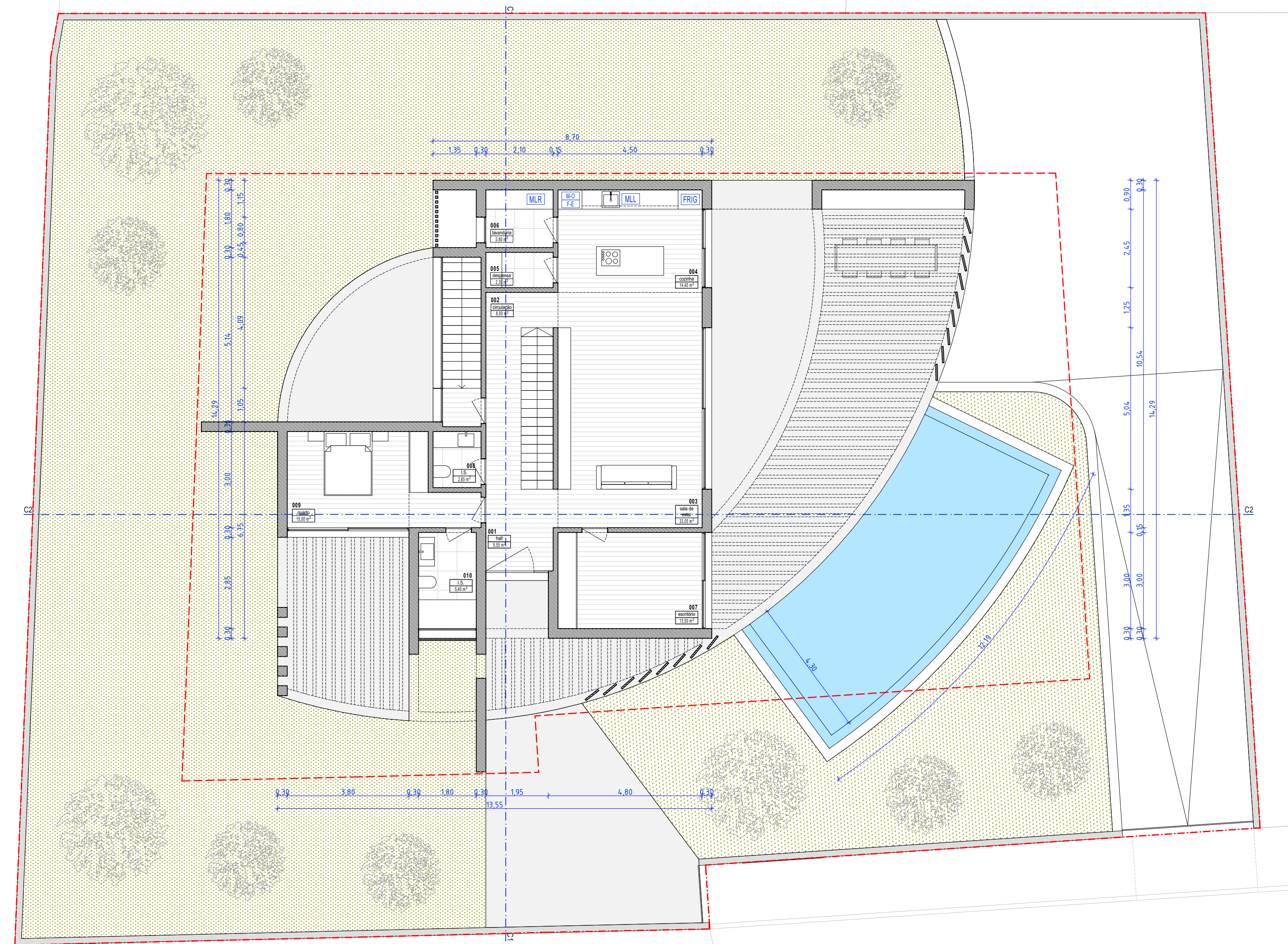
Planta do Piso 0
