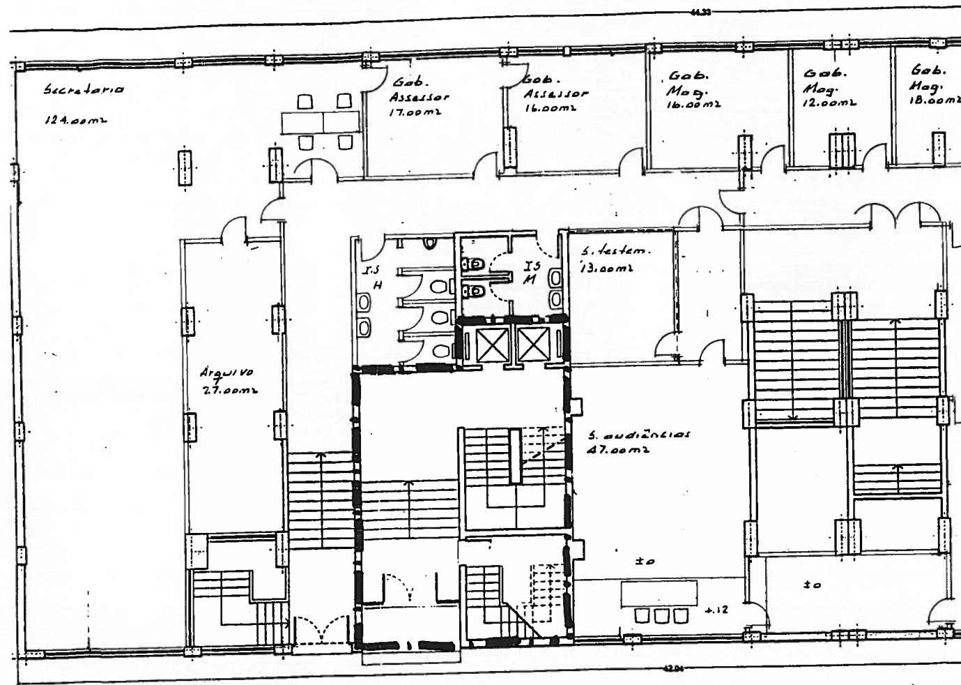
PLANTA DO RÉS-DO-CHÃO - ÁREA = 778m² - ESC. 1/100
