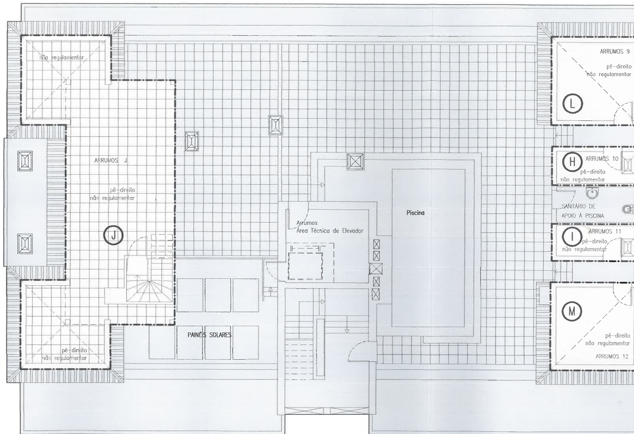
PLANTA DO TERRAÇO/COBERTURA
