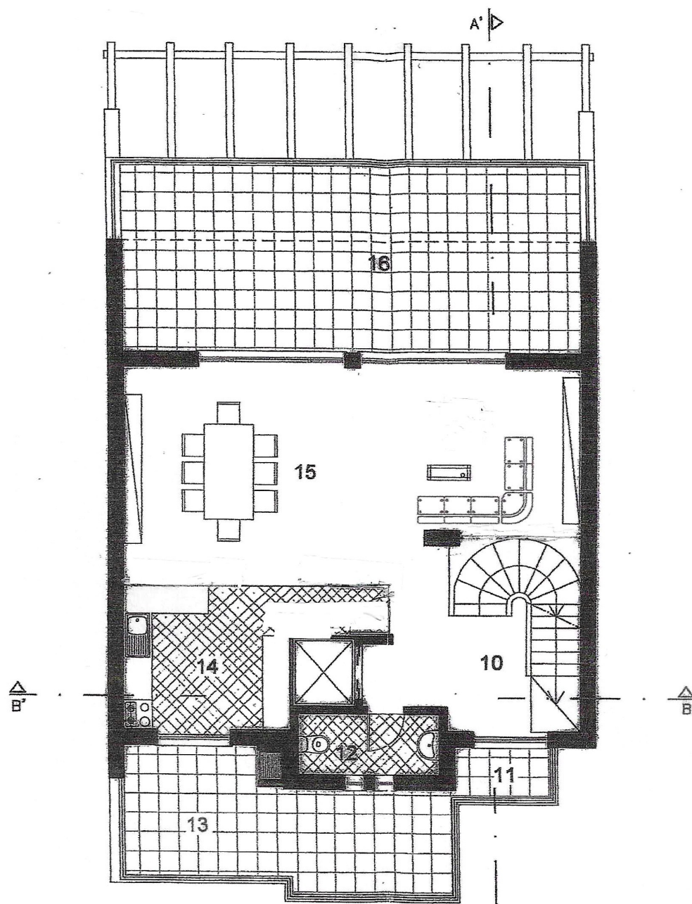
Planta do 1.º Andar
