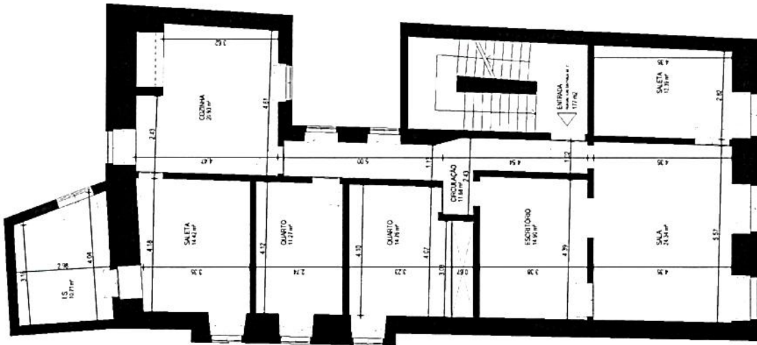
Planta Cotada ESC. 1:100
