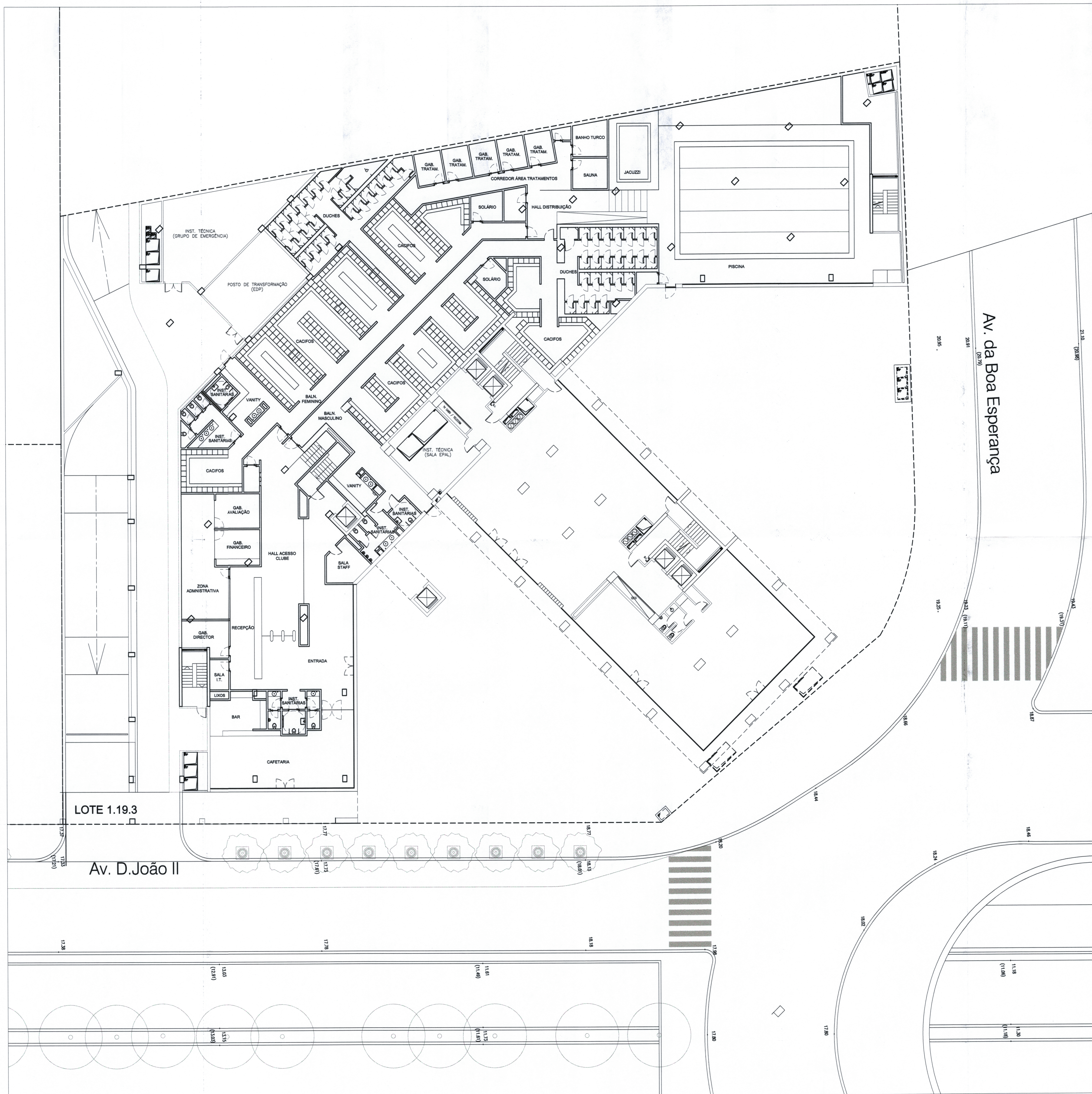
PLANTA PISO 0 ESCALA 1/200
