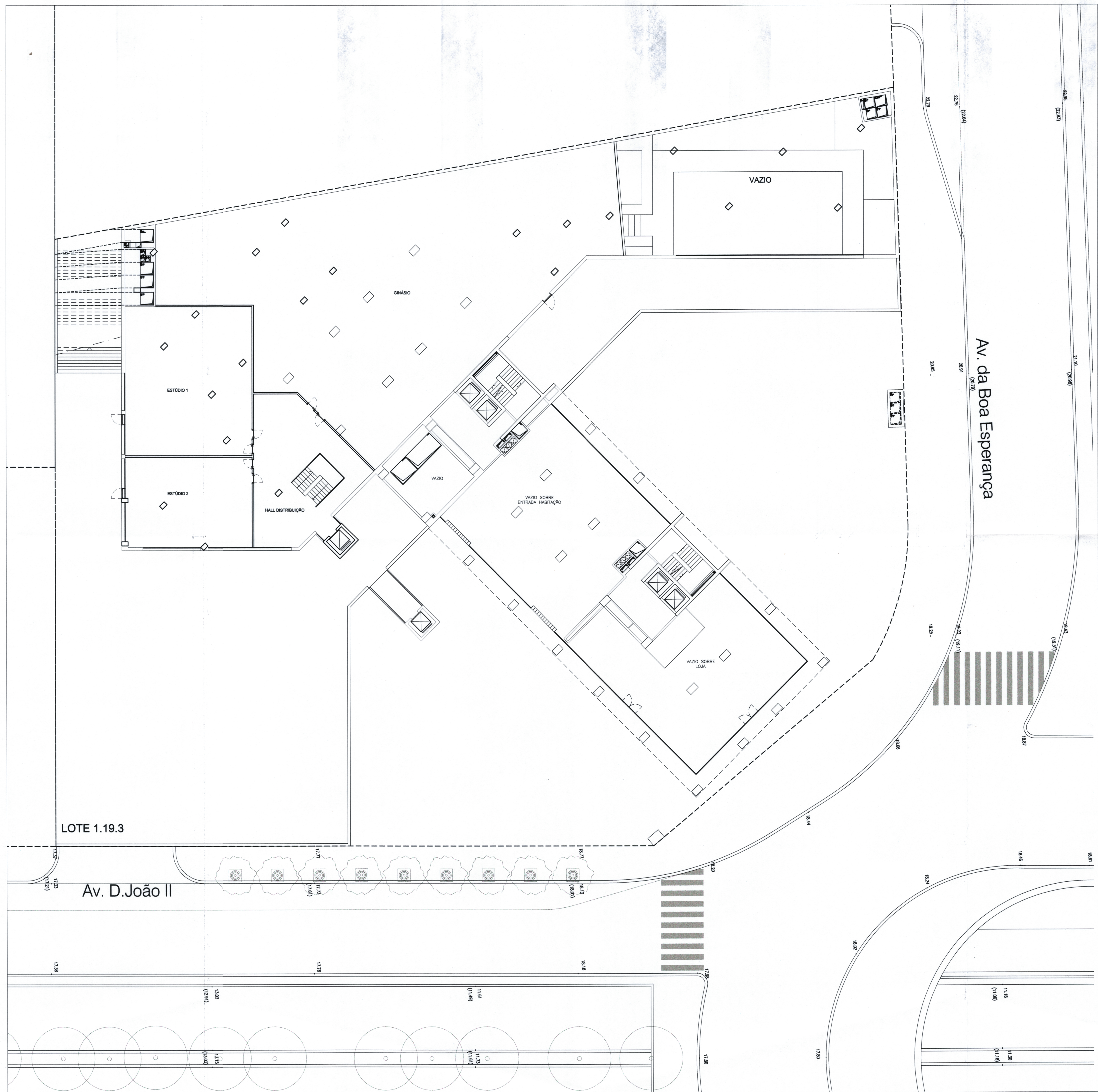
PLANTA PISO 2 ESCALA 1/200
