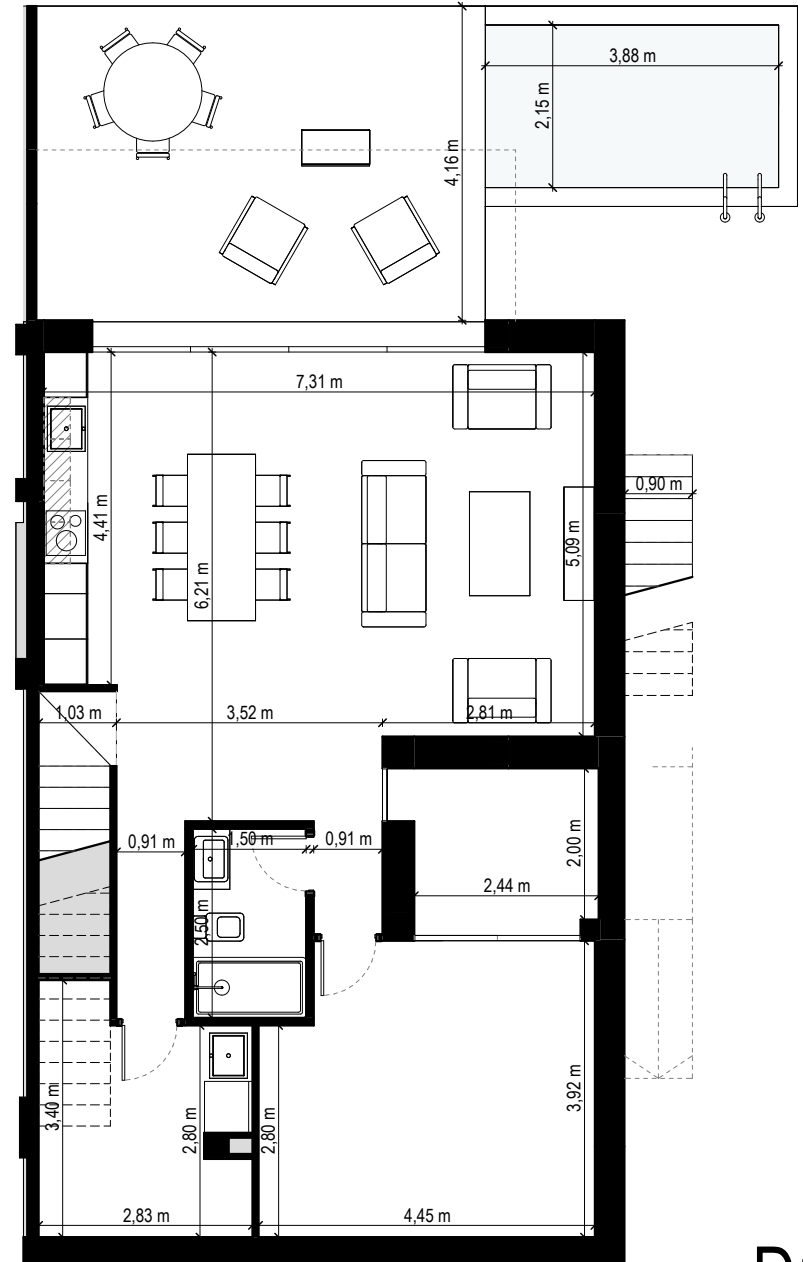
PLANTA BAJA 1 : 100
