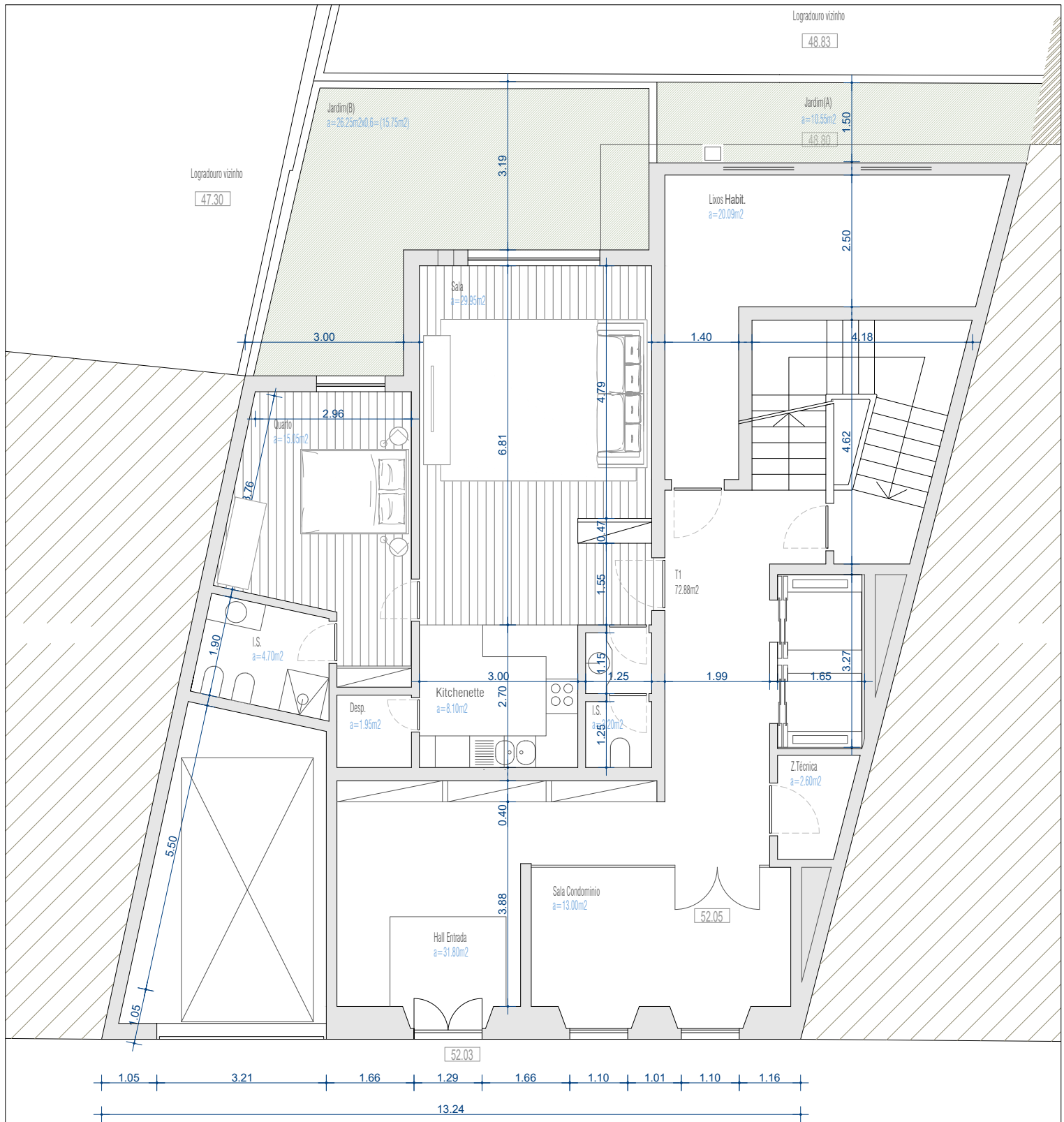
planta piso 0
