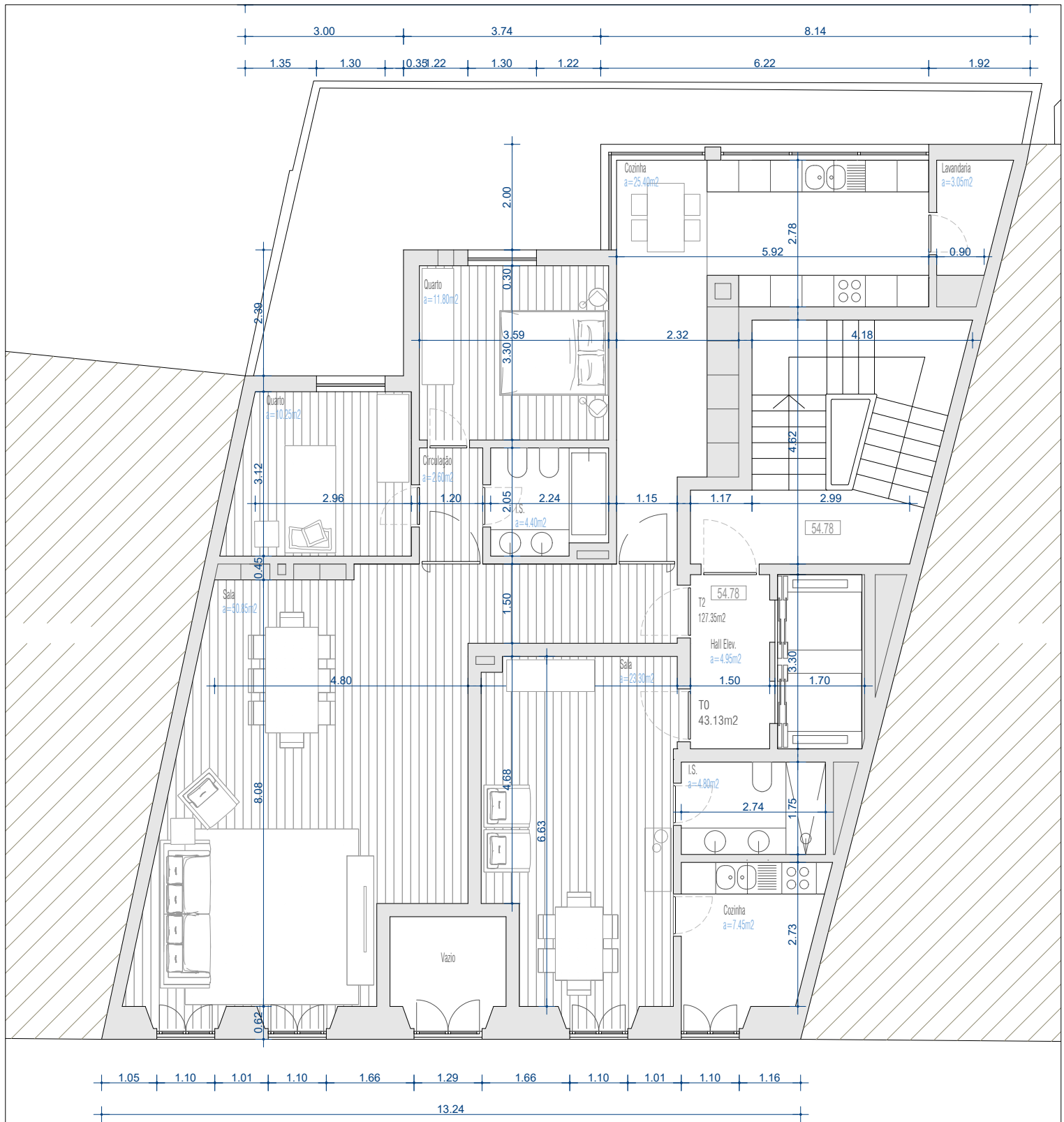
planta piso 1
