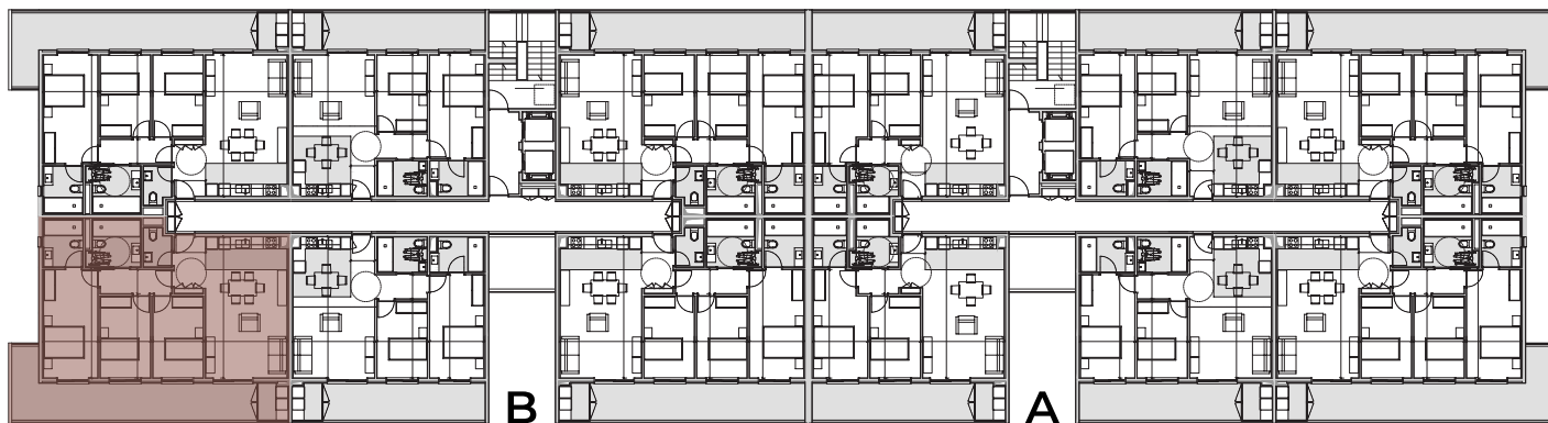
PLANTA DOS PISOS 1, 2, 3, 4, 5, 6
