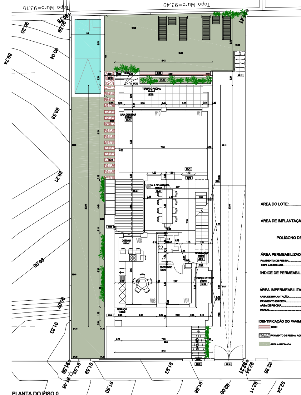
PLANTA DO PISO 0
