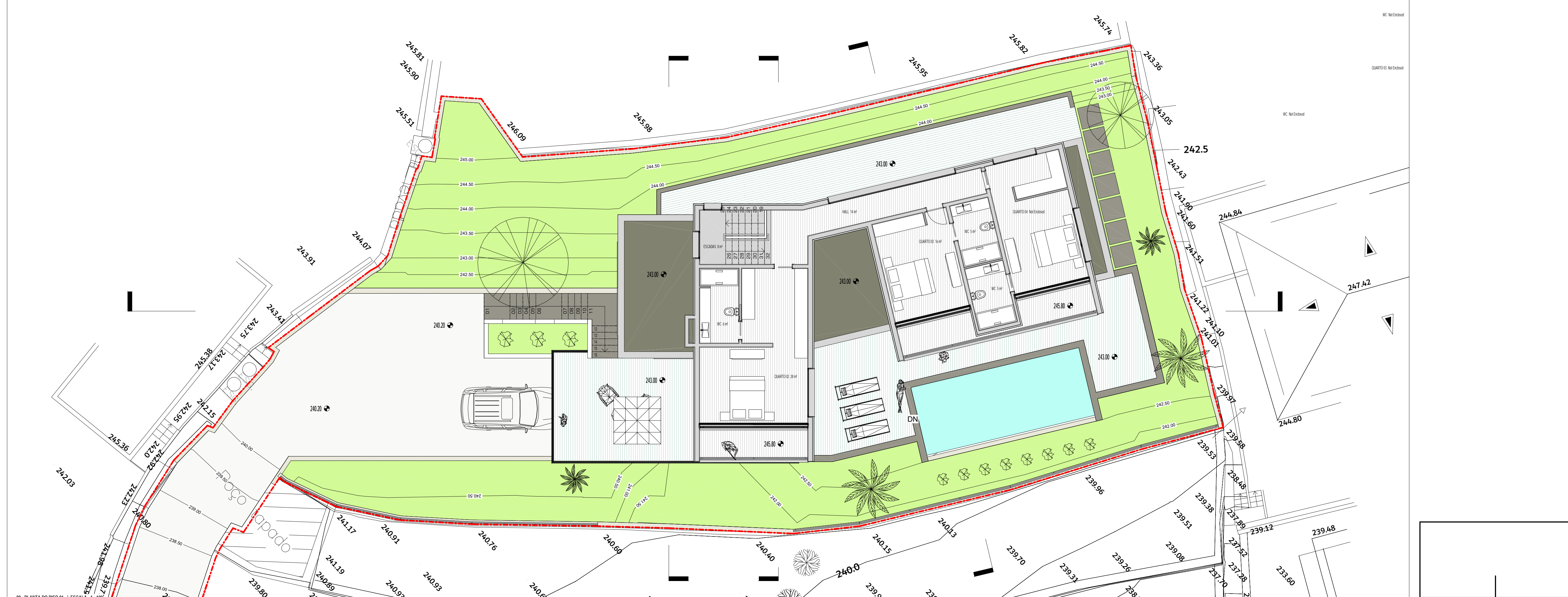
00 - PLANTA DO PISO 01 - ESCALA 1:100
