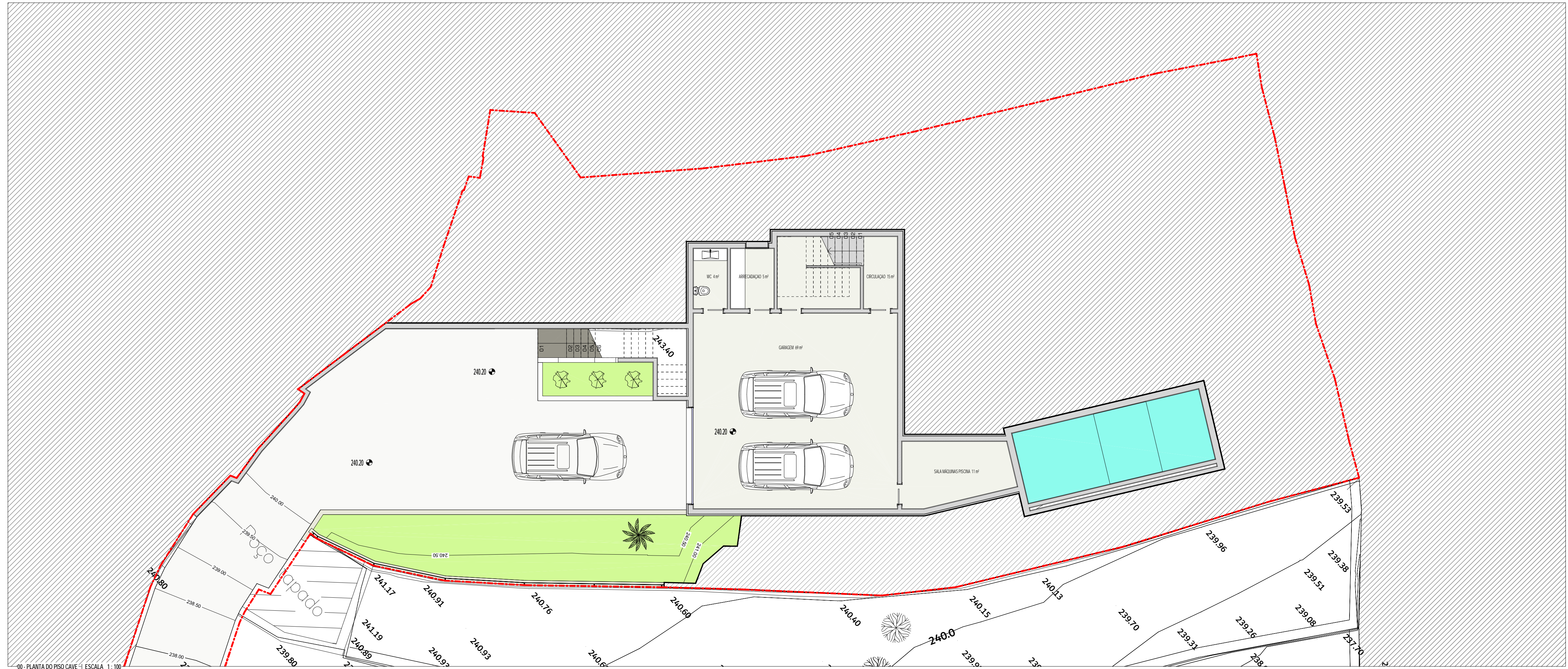
00 - PLANTA DO PISO CAVE | ESCALA 1:100
