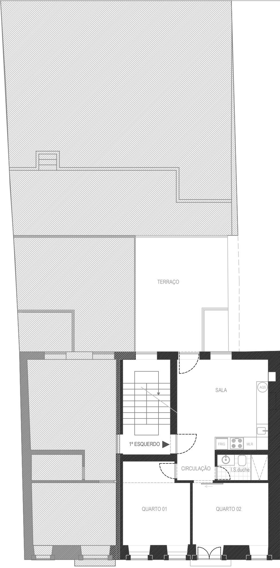
Anexo 6 Planta Simplificada do Fogo
