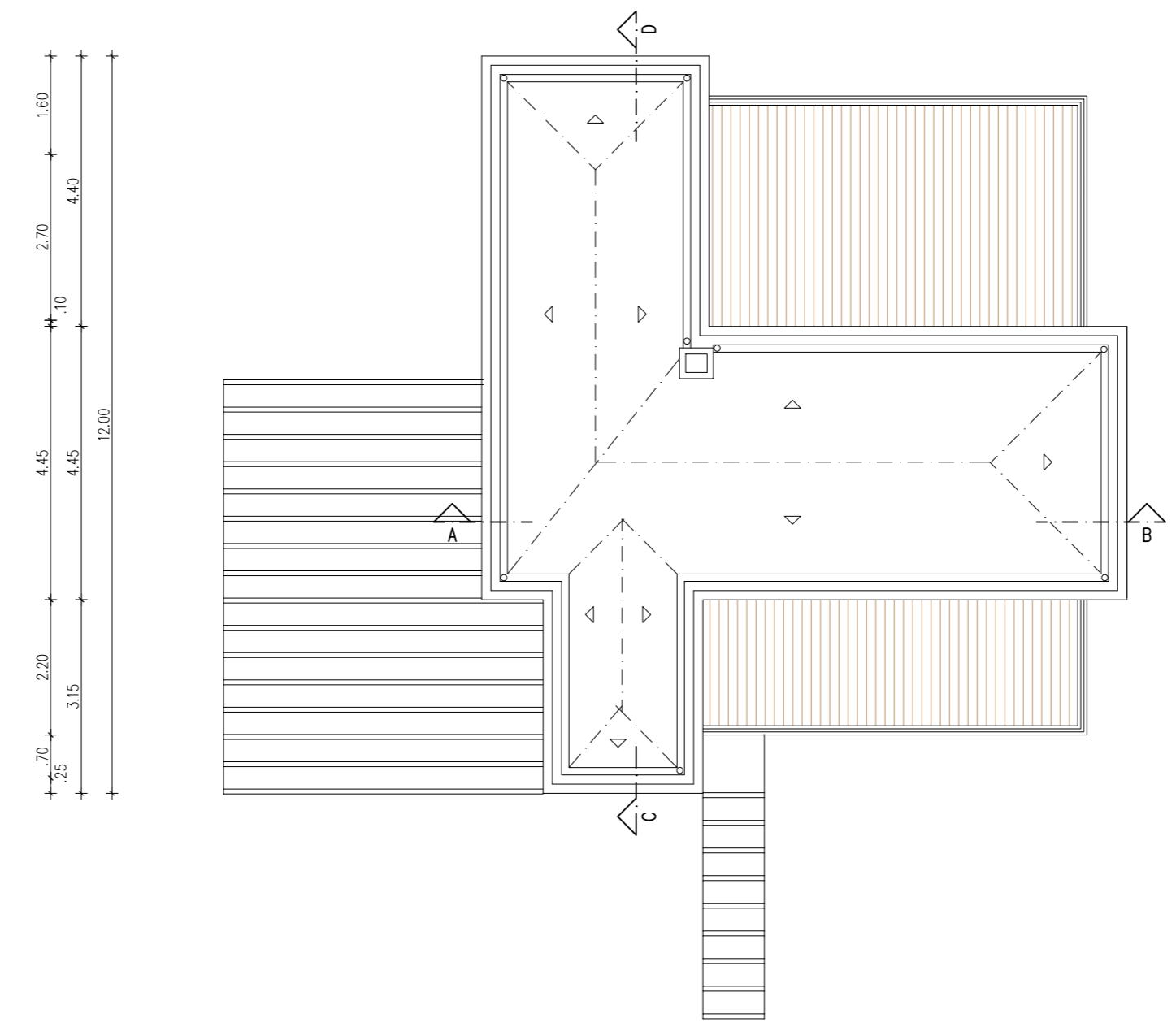
Planta da Cobertura
