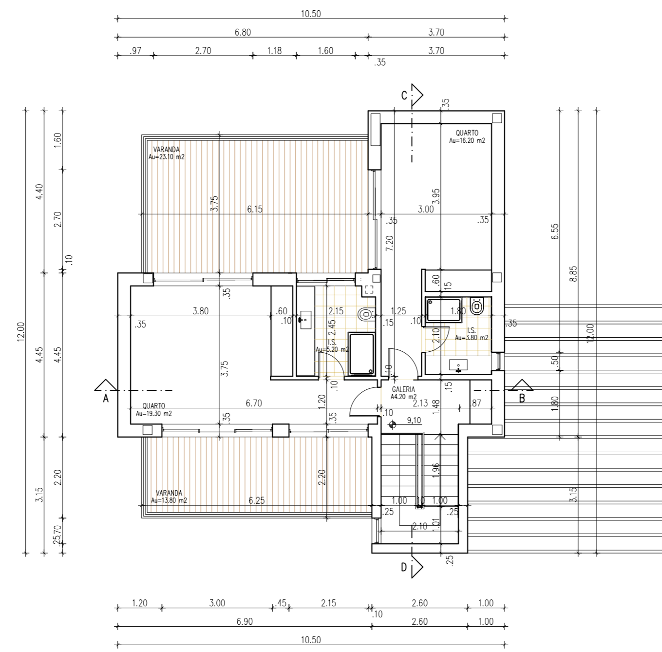
Planta do Piso 1
