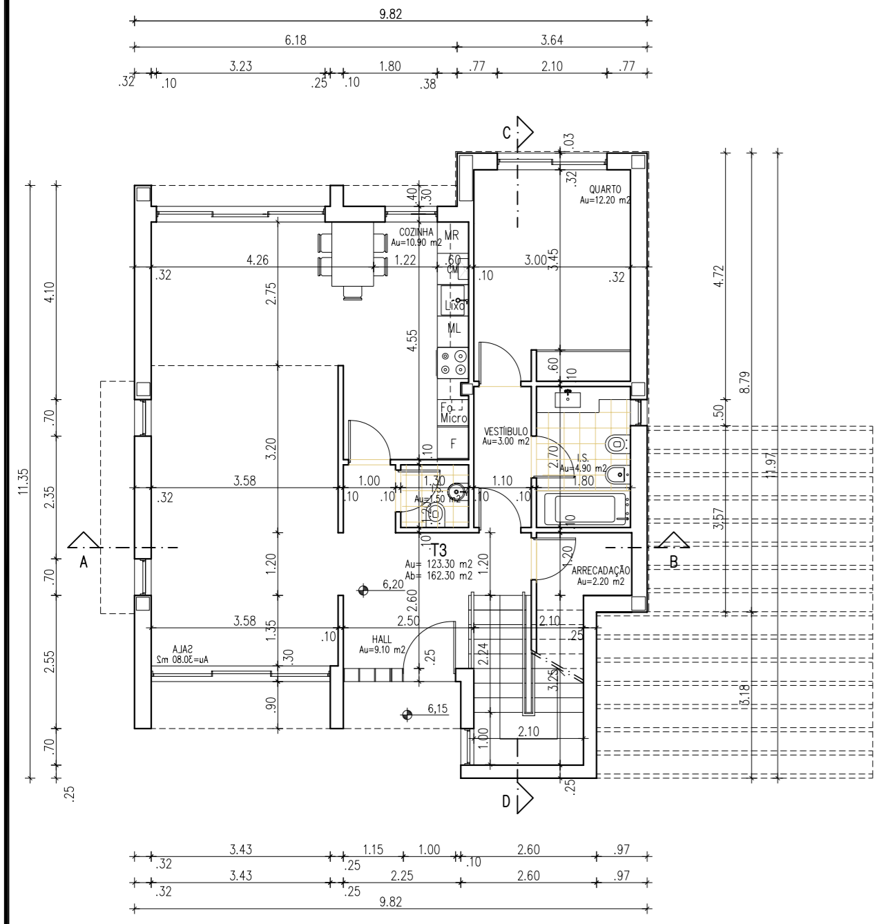
Planta do Piso 0
