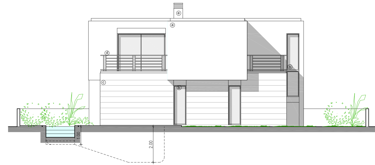
Alçado Poente
