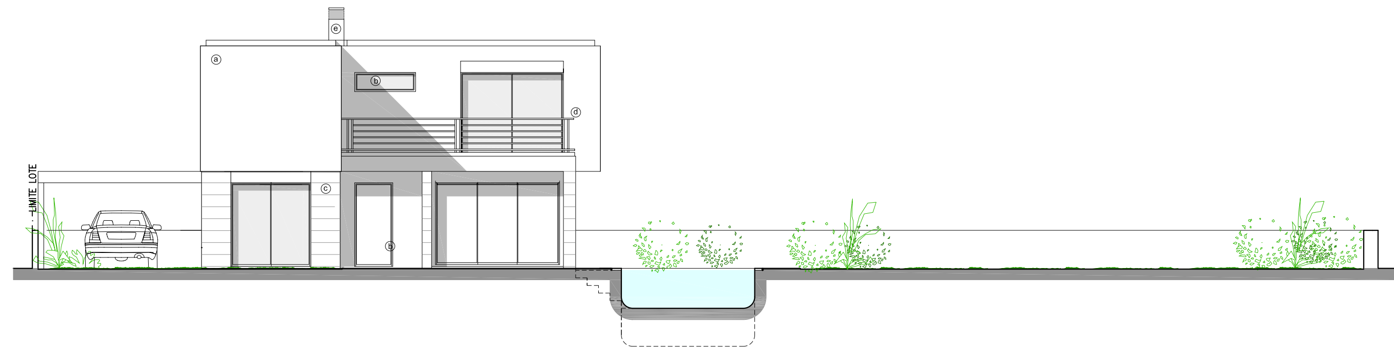
Alçado Sul
