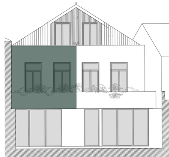
ALÇADO PRINCIPAL
